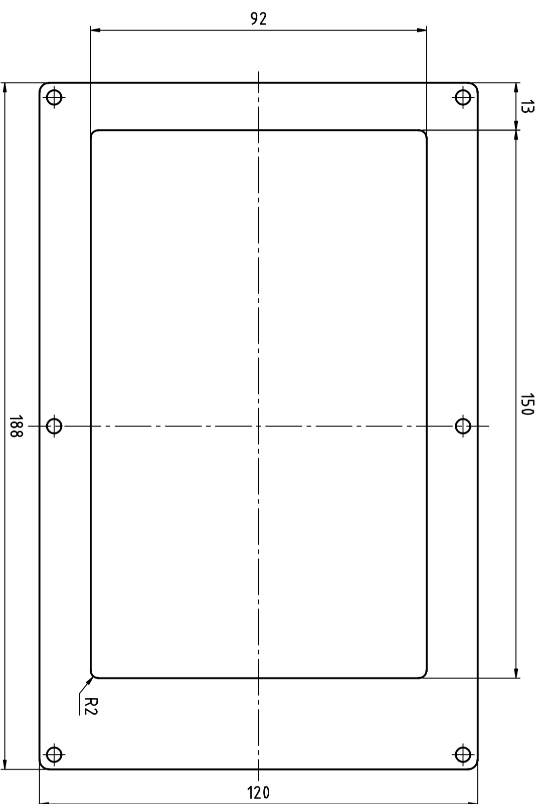
Draufsicht Deckel
